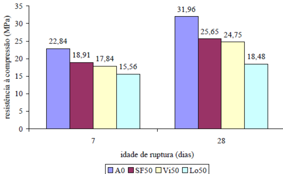
Figura 1: Resultados de resistência á compressão.
